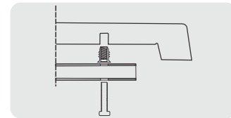
1. Werzalit Table Top 2. M6 Stell Insert
